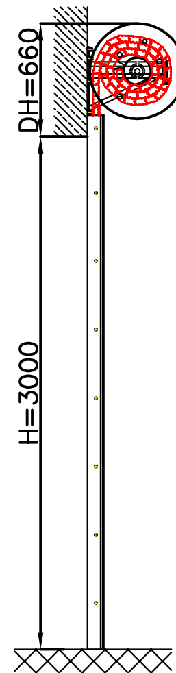
Brama otwarta
